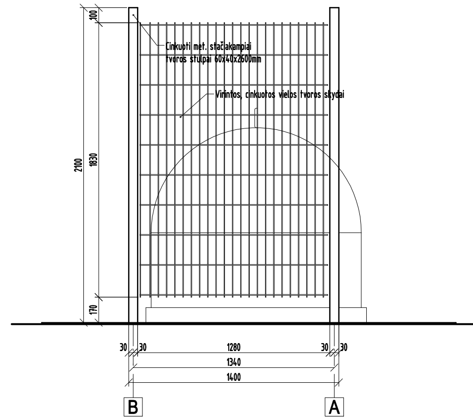
BUITINIŲ ATLIEKŲ AIKŠTELĖ V01. FASADAS TARP AŠIŲ B-A M 1:20
