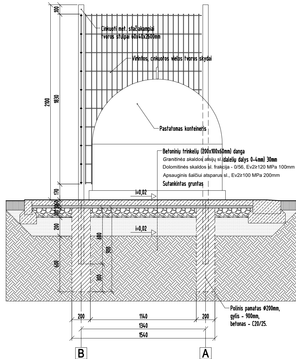
BUITINIŲ ATLIEKŲ AIKŠTELĖ V01. PJŪVIS A-A M 1:20
