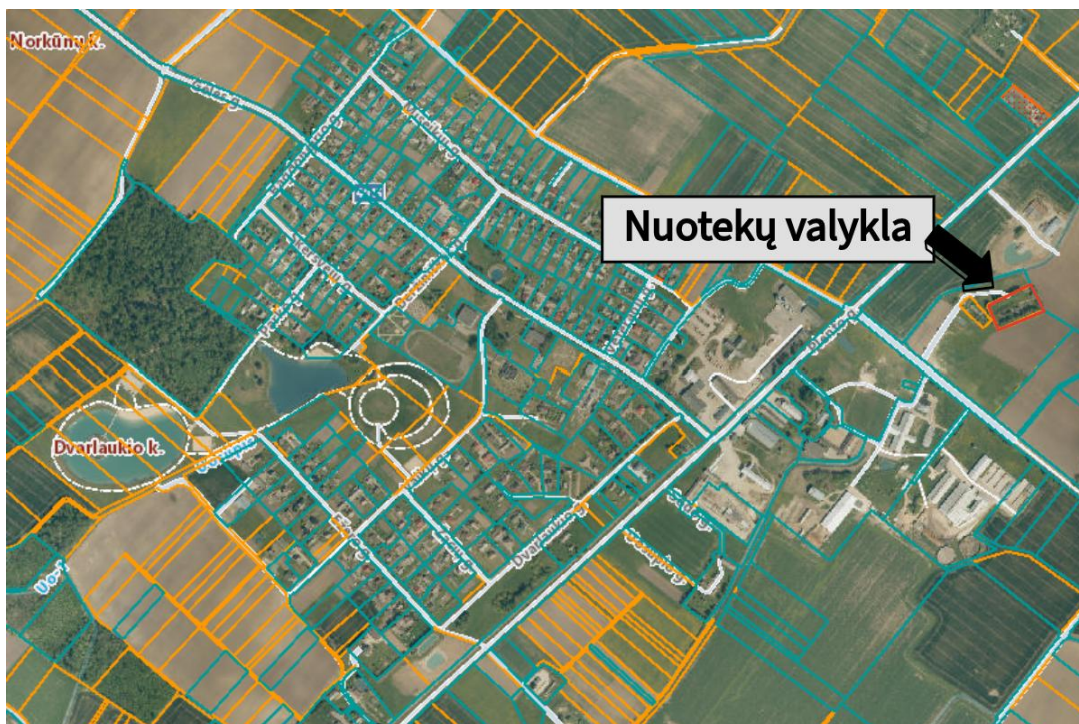
1 pav. Naisių k. NVĮ situacijos schema
