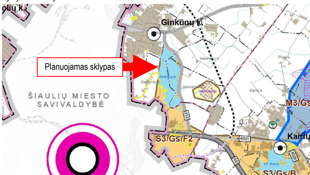
Ištrauka iš Šiaulių rajono savivaldybės teritorijos bendrojo plano keitimo „Gamtinio karkaso sistemos vystymo brėžinys“ brėžinio
